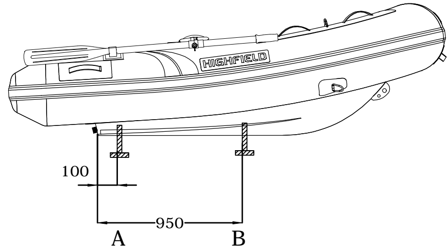
LONGITUDINAL PROFILE
