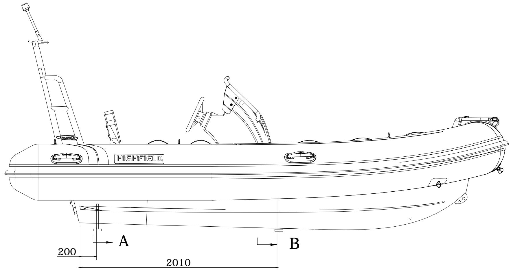
LONGITUDINAL PROFILE
